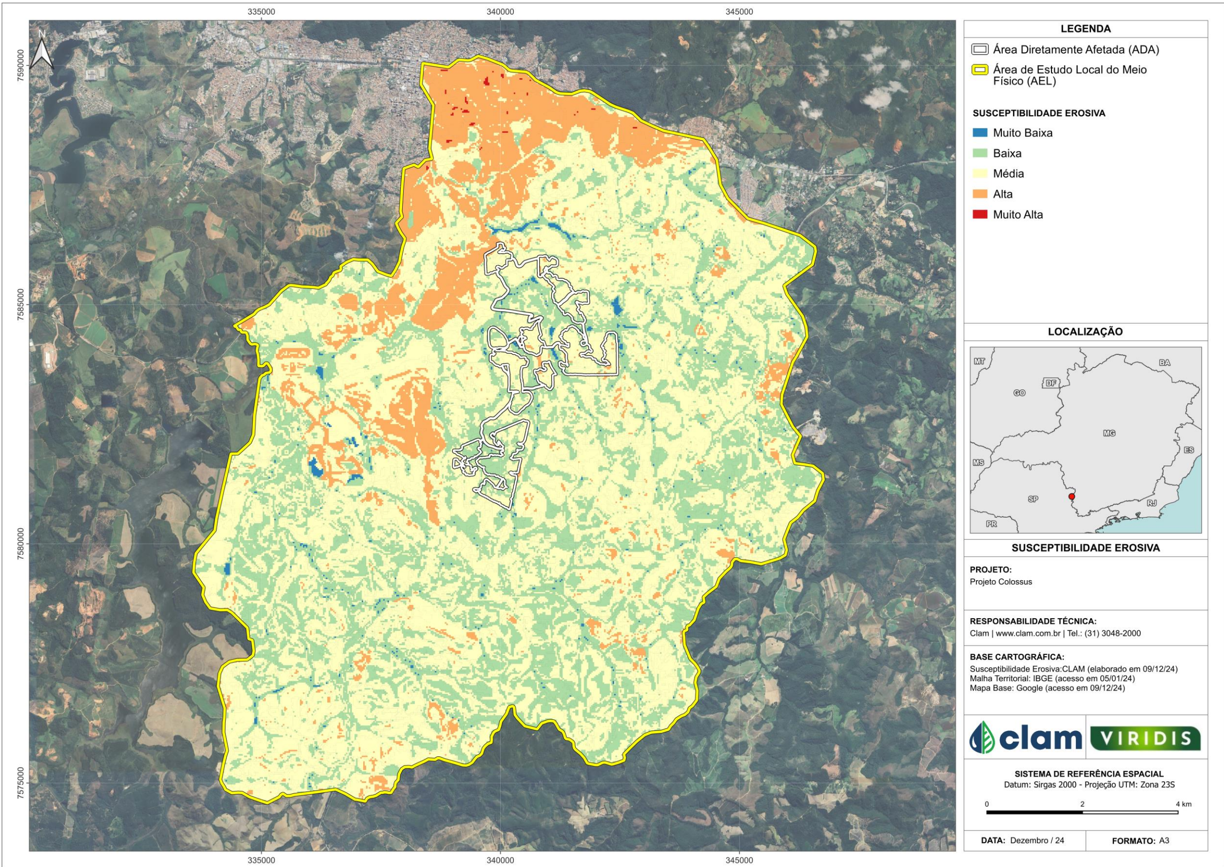
Figura 44 Susceptibilidade erosiva na AEL.
