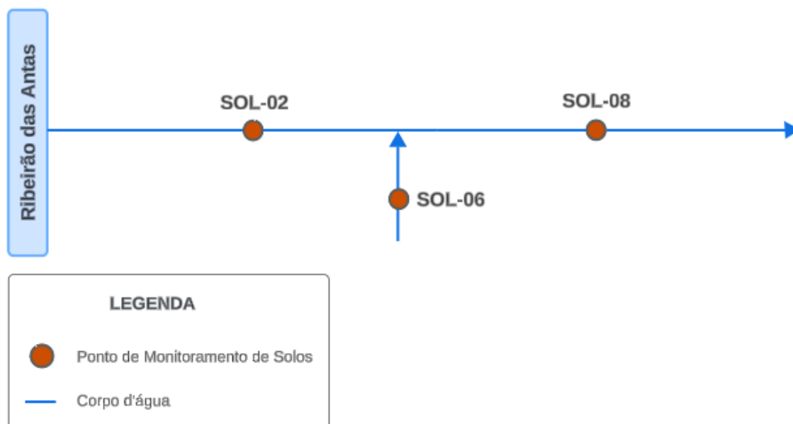
Figura 235 Diagrama unifilar da sub-bacia hidrográfica do ribeirão das Antas
